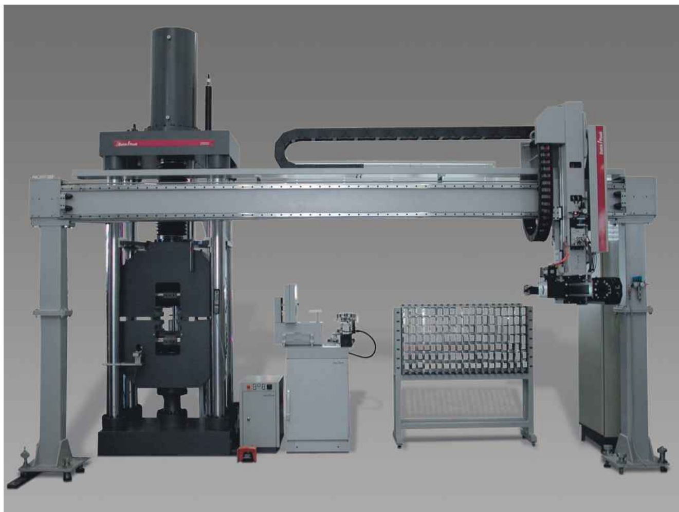
Рис.1: Автоматизированное испытание толстолистового проката на растяжение (система roboTest B)
