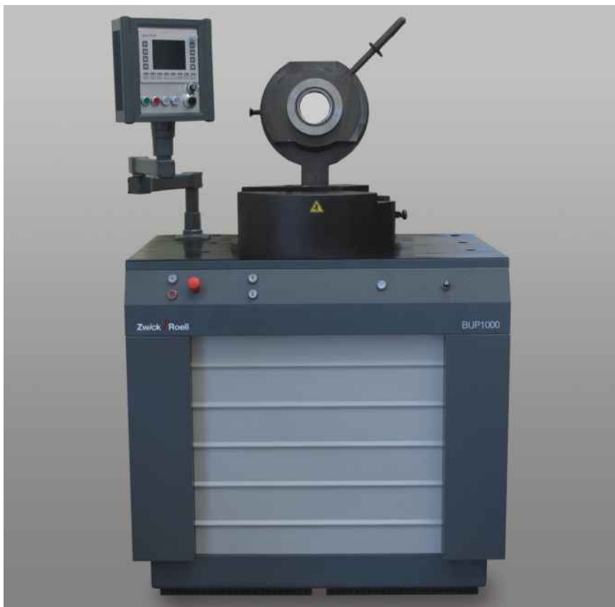
Рис.2: Машина для испытаний на глубокую вытяжку BUP 1000
