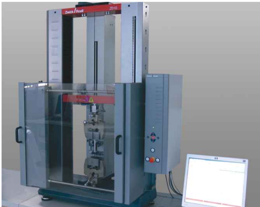
Рис.2: Машина ProLine Z050TN с защитным приспособлением
