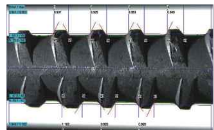
Рис.6: Автоматический промер рифлений
