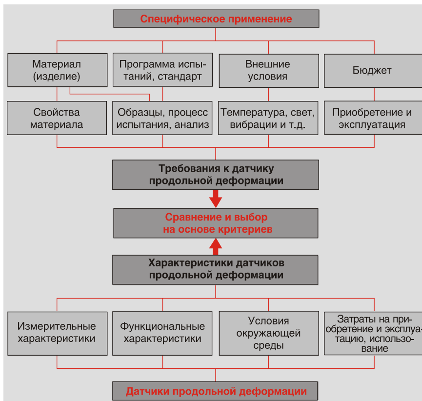
Рис.1: Процесс выбора датчиков продольной деформации
