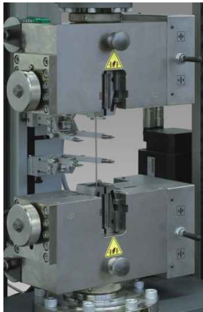
Рис.1: Испытание тонкой проволоки на растяжение с датчиком продольной деформации Макро
