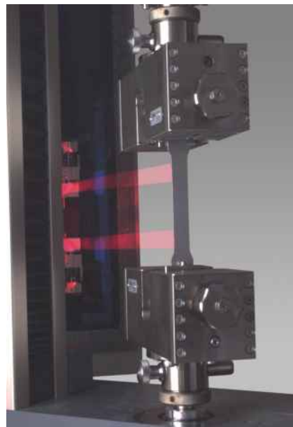
Рис.4: Датчик optiXtens
