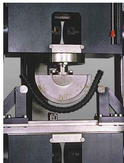
Рис.2: Приспособление для испытаний рифленой арматурной стали на изгиб
