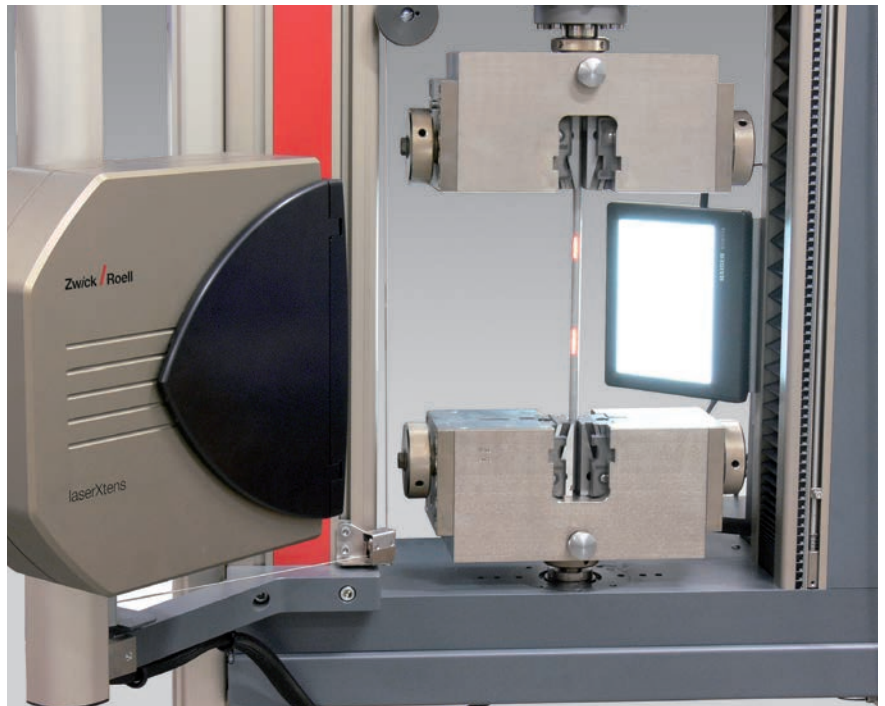
Bild 1: Längenänderungsaufnehmer laserXtens mit Option videoXtens für Breitenänderung
