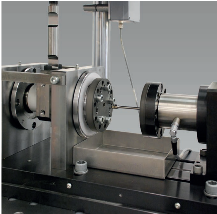
Bild 2: Torsionsprüfvorrichtung für Hochfrequenzpulsator Vibrophore
