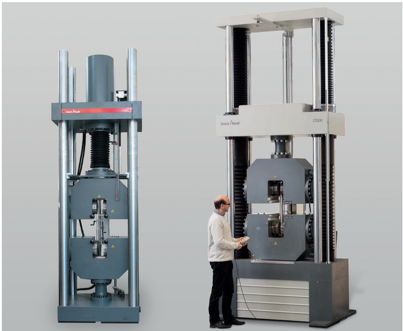
Bild 1: ZwickRoell bietet standardmäßig Großlast-Prüfmaschinen bis 2.500 kN
