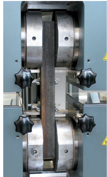
Bild 3: Zugversuch an Rohrwandprobe
