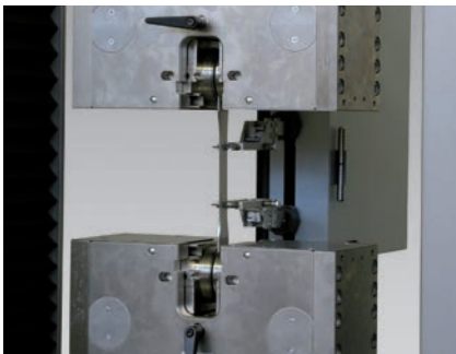
Bild 3: Pneumatik-Probenhalter, Probenhalter für Schrauben, Schulter- und Gewindekopfproben, Hochtemperatur-Probenhalter
