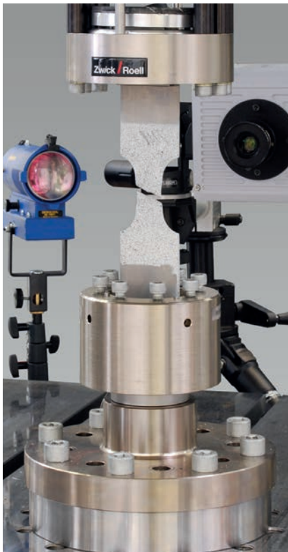
Bild 1: Metallprobe in Schnellzerrei-Prfmaschine HTM
