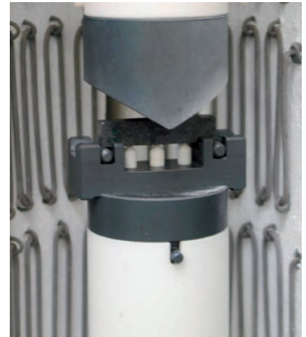
Bild 3: Warmbiegeversuch im Hochtemperaturofen
