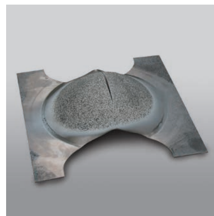
Bild 4: Probe aus FLC-Versuch (Nakajima)
