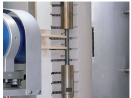
Bild 3: Pneumatik-Probenhalter, Probenhalter für Schrauben, Schulter- und Gewindekopfproben, Hochtemperatur-Probenhalter
