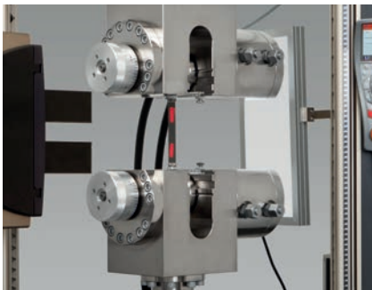
Bild 2: Hydraulik-Probenhalter, Hydraulik-Probenhalter (Körper über Keil), Kurzspannender Hydraulik-Probenhalter
