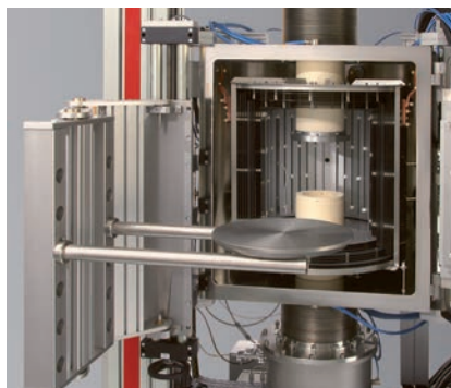
Bild 4: Hochtemperaturversuche im Vakuum-Ofen
