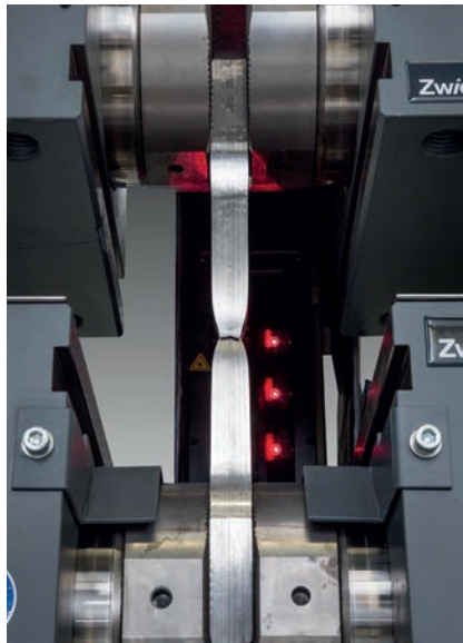
Bild 1: Grobblech Probe mit Längenänderungsaufnehmer laserXtens
