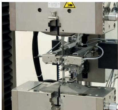
Bild 1: makroXtens und Variante mit optionaler Feindehnungsmessung (unten)
