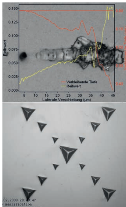
Bild 2: Scratchtest und Berkovich-Eindrücke
