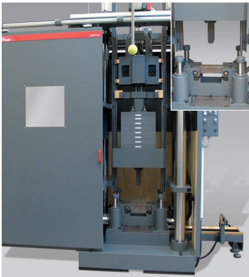
Bild 2: Probe in Großfallwerk DWT
