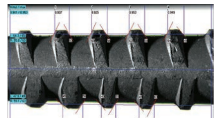
Bild 6: Automatische Rippenvermessung
