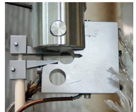
Bild 2: Rissaufweitungs- und Rissfortschrittsmessung nach ASTM E 1457
