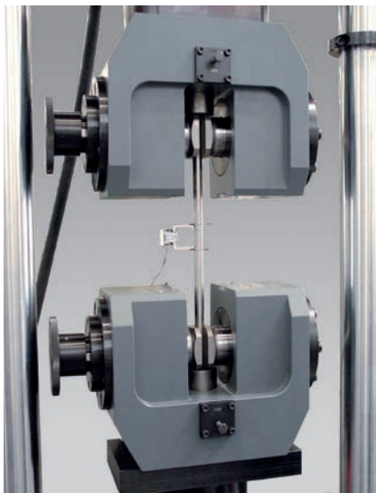
Bild 1: Ermüdungsversuch an Rundprobe
