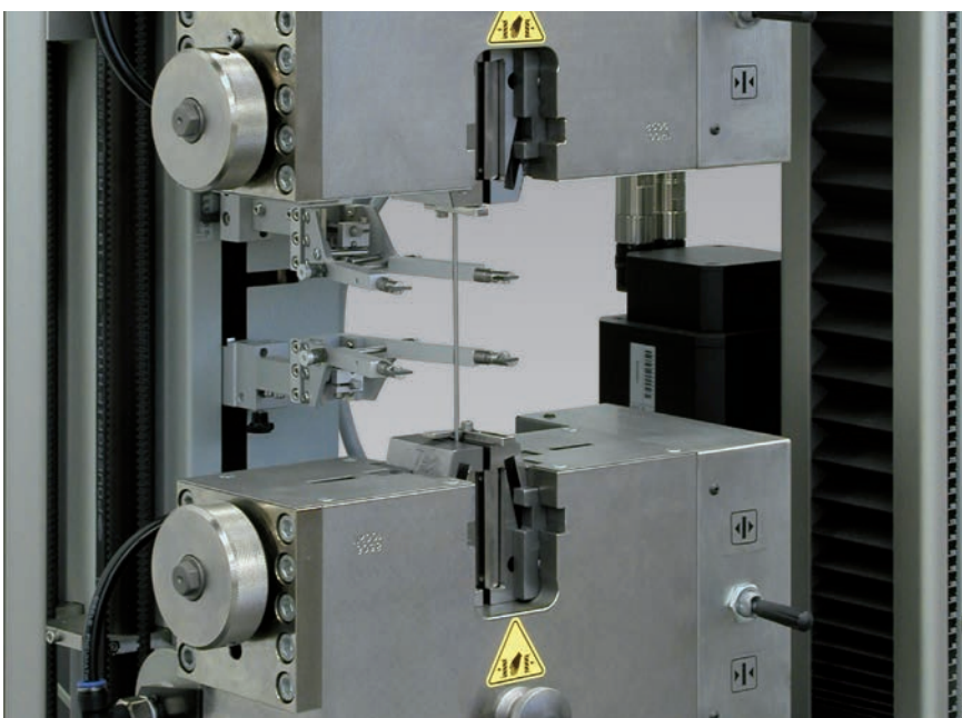
Bild 1: Zugversuch an Feindraht mit Längenänderungsaufnehmer makroXtens
