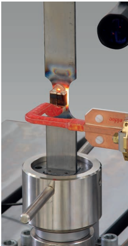
Bild 2: Schnellzerreiversuch unter Hochtemperatur
