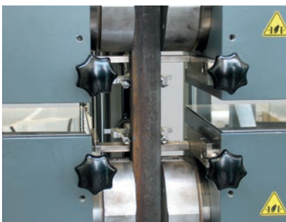
Bild 4: Hydraulische Großlast-Probenhalter für Prüfanwendungen bis 2.500 kN
