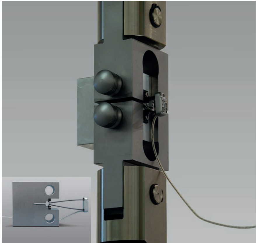
Bild 1: CT Probe in Hochfrequenzpulsator Vibrophore
