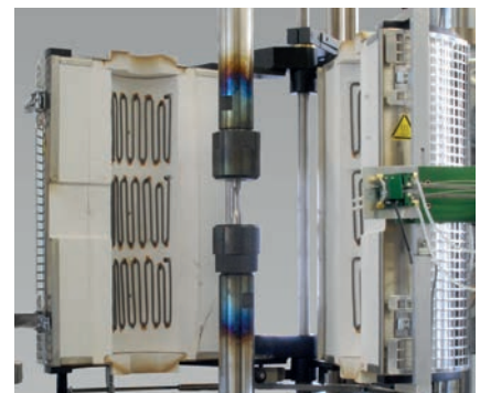
Bild 6: Servohydraulische Prüfmaschine mit Hochtemperatur-Ofen
