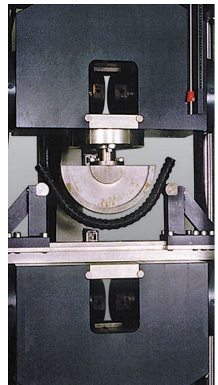
Bild 2: Biegevorrichtung für Betonrippenstahl, eingebaut in Probenhalter für Zugversuche
