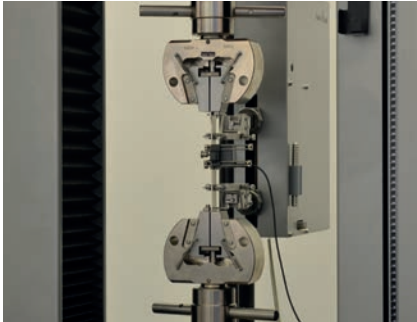
Bild 1: Keil-Probenhalter und Keil-/Keilschraub-Probenhalter
