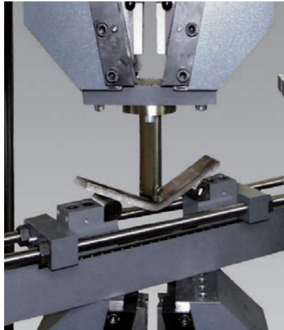
Bild 1: 3-Punkt-Biegeeinrichtung für Blechstreifen
