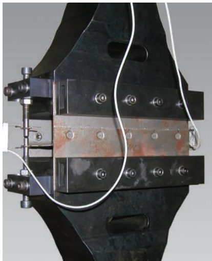
Bild 2: Ermüdungsprüfung an H-Proben
