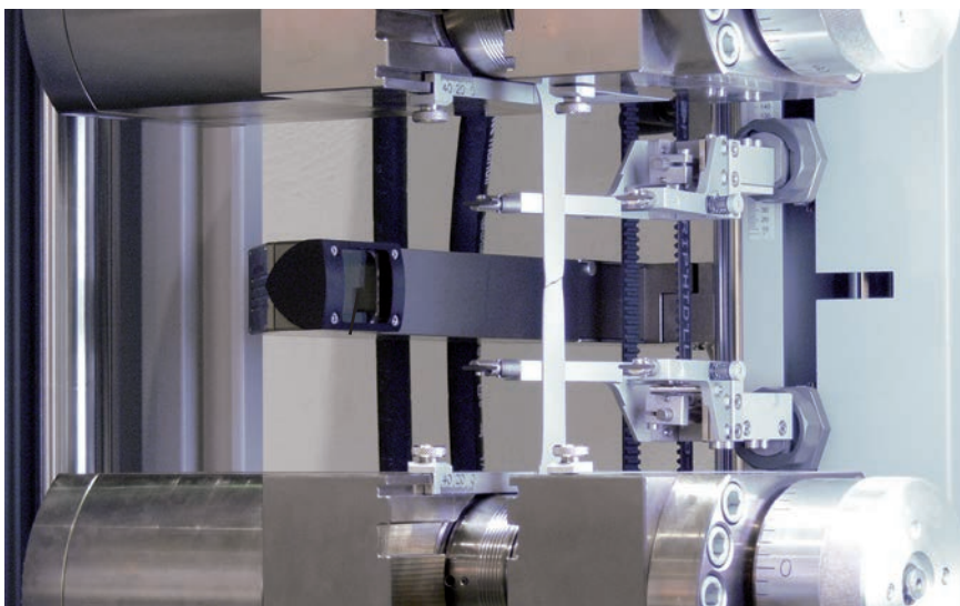
Bild 1: Breitenänderungsaufnehmer videoXtens und Längenänderungsaufnehmer makroXtens
