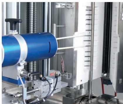
Bild 2: Hochtemperatur-Ofen mit HT-Längenänderungsaufnehmer
