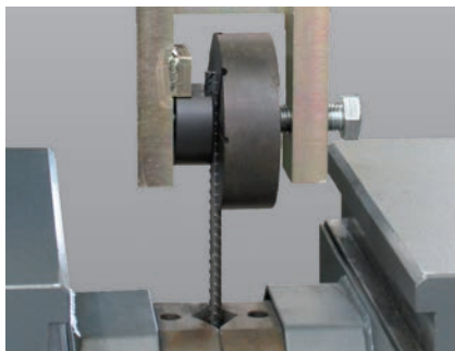
Bild 2: Abscherversuch an Gitterträger
