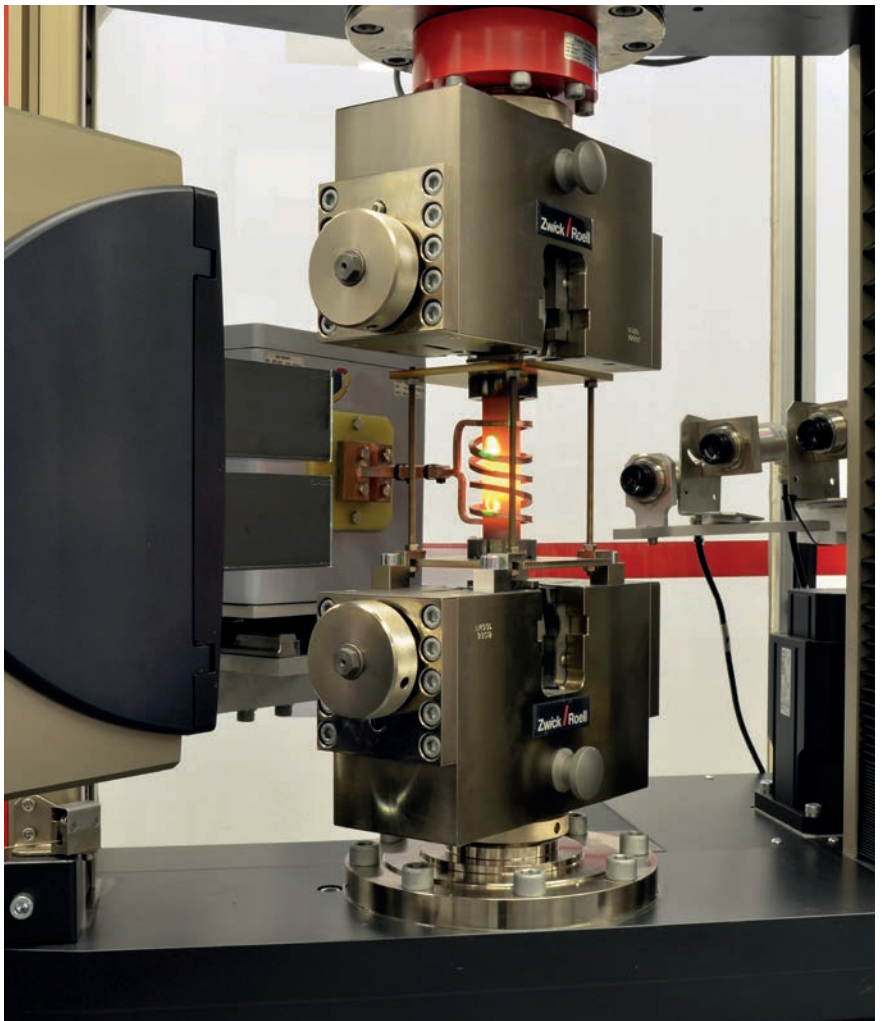
Bild 2: Warmzugversuch mit Induktionsheizung und Längenänderungsaufnehmer laserXtens mit Pyrometer zur Temperaturmessung
