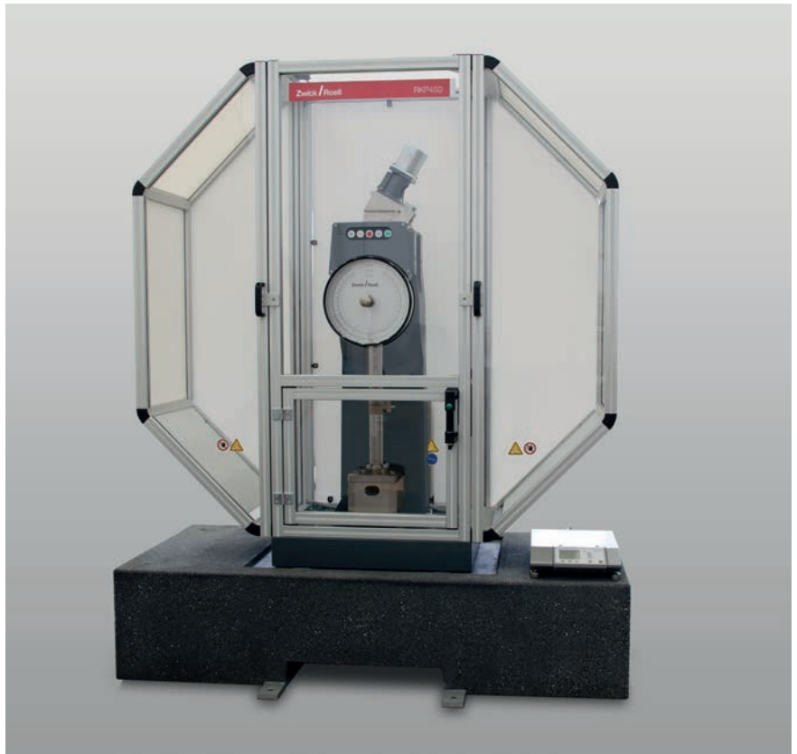
Bild 1: Pendelschlagwerk RKP 450 mit optionalem Betonsockel
