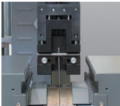
Bild 1: Schweißnahtprüfung an T-Verbindung
