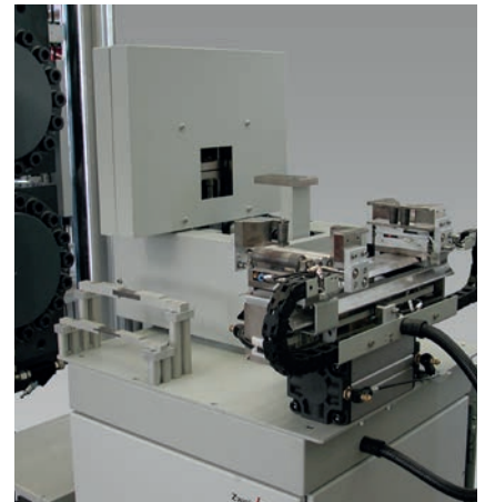
Bild 2: Automatisches Querschnittsmessgerät (QMG)
