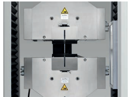
Bild 2: Hydraulik-Probenhalter, Hydraulik-Probenhalter (Körper über Keil), Kurzspannender Hydraulik-Probenhalter
