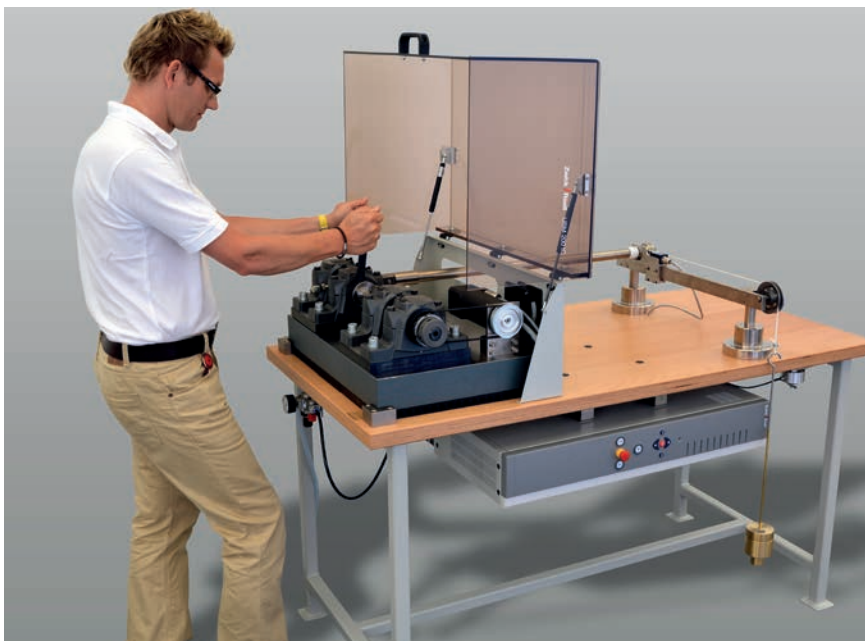
Bild 2: Umlaufbiege-Prüfmaschine UBM
