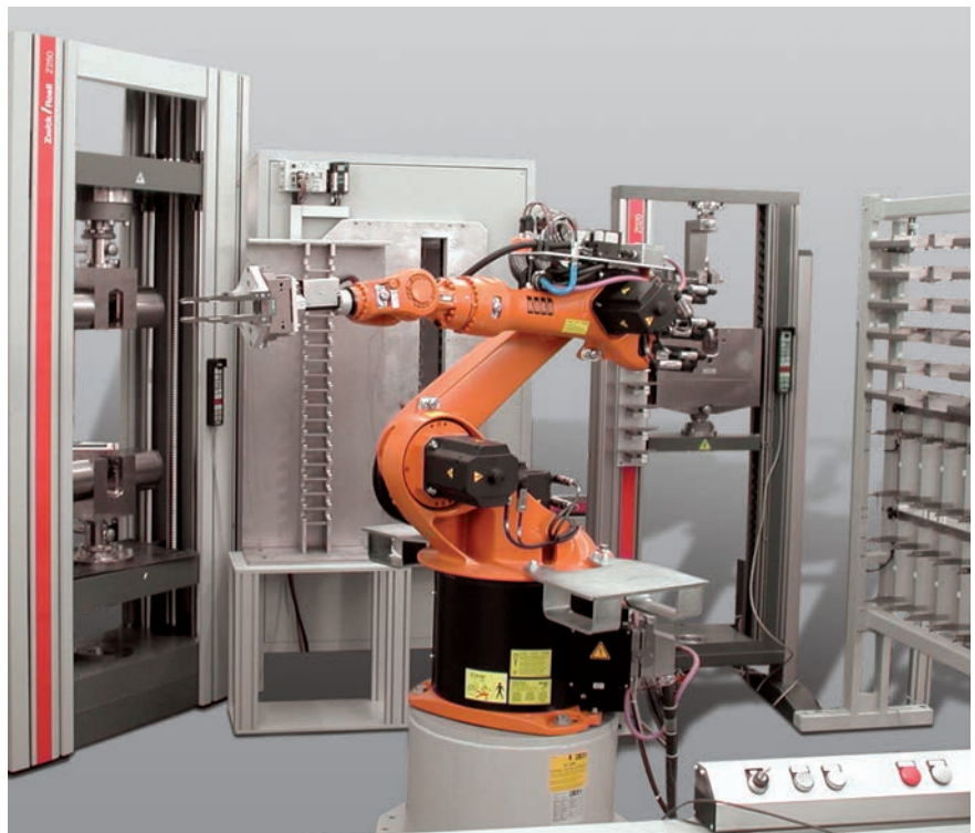
Bild 4: Roboter-Prüfsystem für Betonstahlprüfung roboTest R
