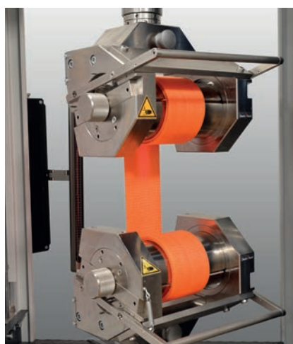
Bild 3: Walzen-Probenhalter
