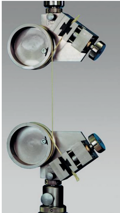
Bild 1: Zugversuch an Multifilamentgarn
