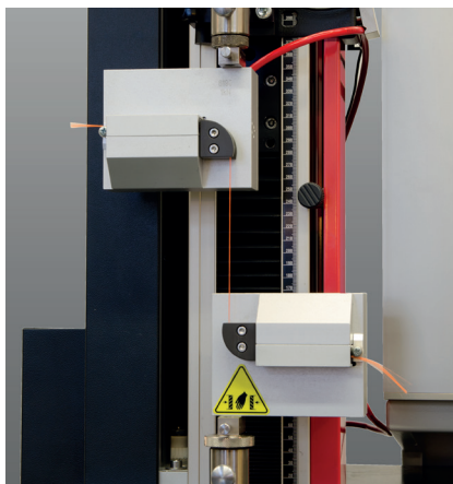
Fig. 2. Capstan grips
