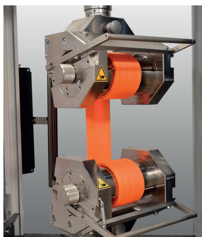
Fig. 3. Roller grips
