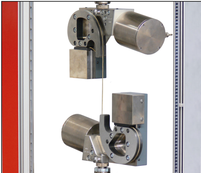
Umlenk-Probenhalter für Stahlreifencorde nach BISFA Typ 8397, Fmax 10 kN
