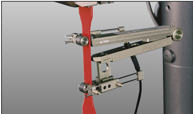
Ansetzaufnehmer, Typ DMS Länge 1 mit Verlängerungsstück
