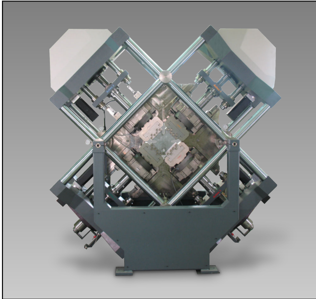
Kreuzzug-Prüfmaschine 250 kN
