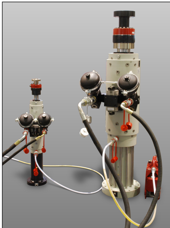
LH-Einzelprüfzylinder mit optionalem Fußflansch
