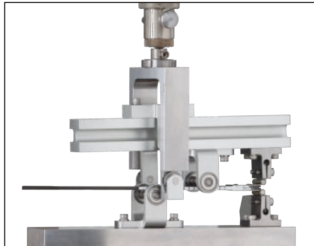
Mixed Mode-Biegevorrichtung
