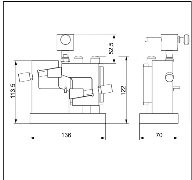
Schervorrichtung Maße
