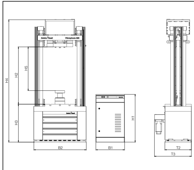
Zeichnung. Vibrophore 250
