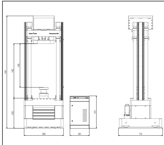
Zeichnung: Vibrophore 600
